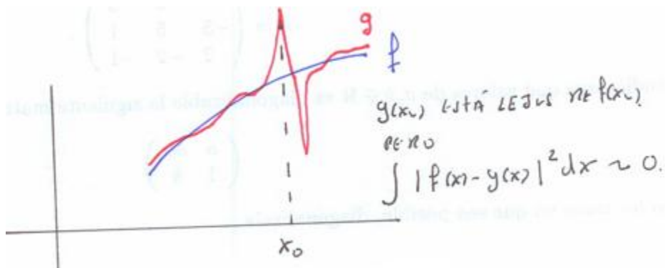
FIGURA 2. Convergencia en media cuadrática
