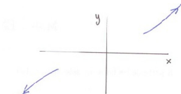
FIGURA 2. Función que se hace muy grande en valor absoluto cuando |x| se hace grande.
