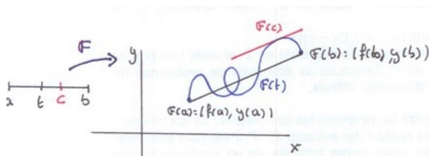
FIGURA 4. Teorema del Valor Medio de Cauchy.
