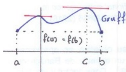
FIGURA 1. Teorema de Rolle.
