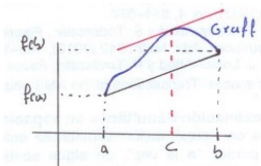
FIGURA 2. Teorema del Valor Medio.
