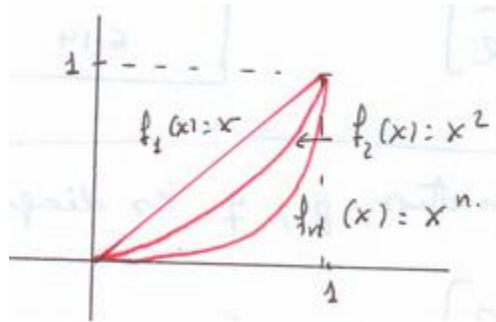
FIGURA 3. Gráficas de f_1, f_2, \dots, f_n
