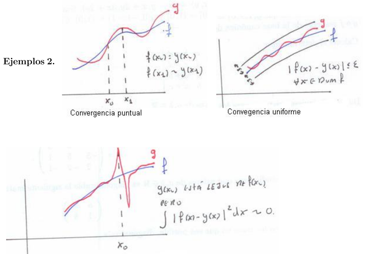
FIGURA 2. Convergencia en media cuadrática
