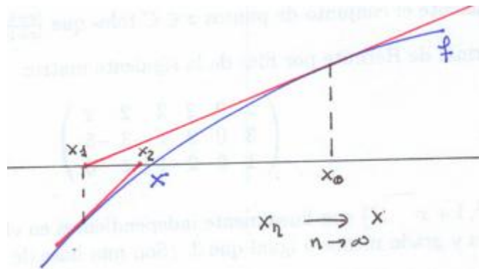
FIGURA 1. Tangentes de Newton
