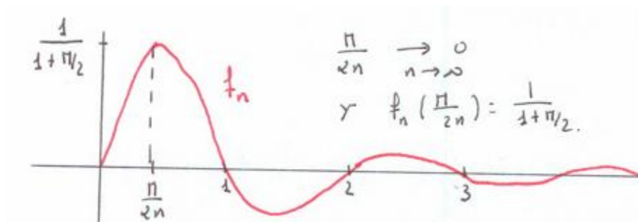
FIGURA 5. Gráfica de f_n
